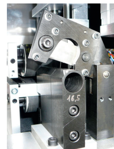
Schlauchschneideeinheit
